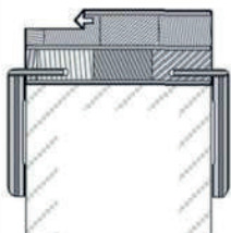
Telaio Spigolo con guarnizione Frame Spigolo with gasket Cadre Spigolo avec garniture
