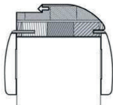
Telaio Round con guarnizione Frame Round with gasket Cadre Round avec garniture
